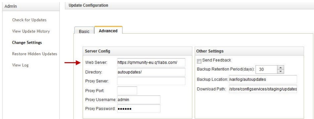
Figure 1. Mise à jour de l'adresse du serveur de mise à jour automatique QRadar
